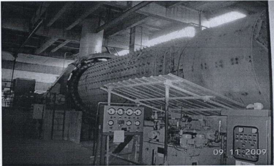
ຮູບ 3: ປັດວັດຖຸດິບໃຫ້ເປັນແປ້ງ
